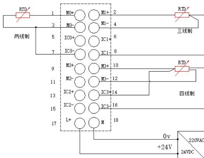
接线图
