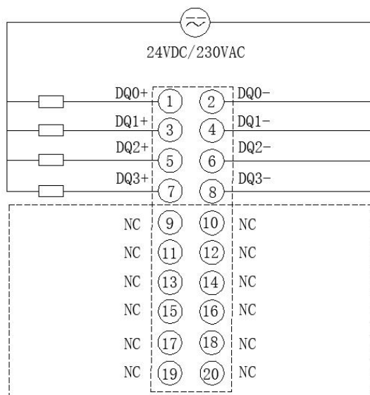
接线图
