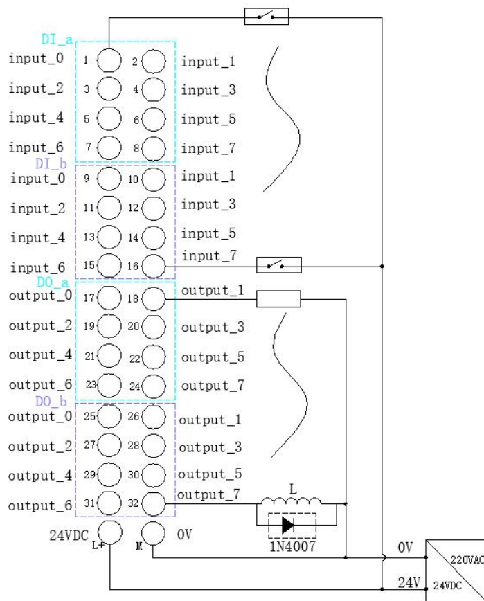
接线图
