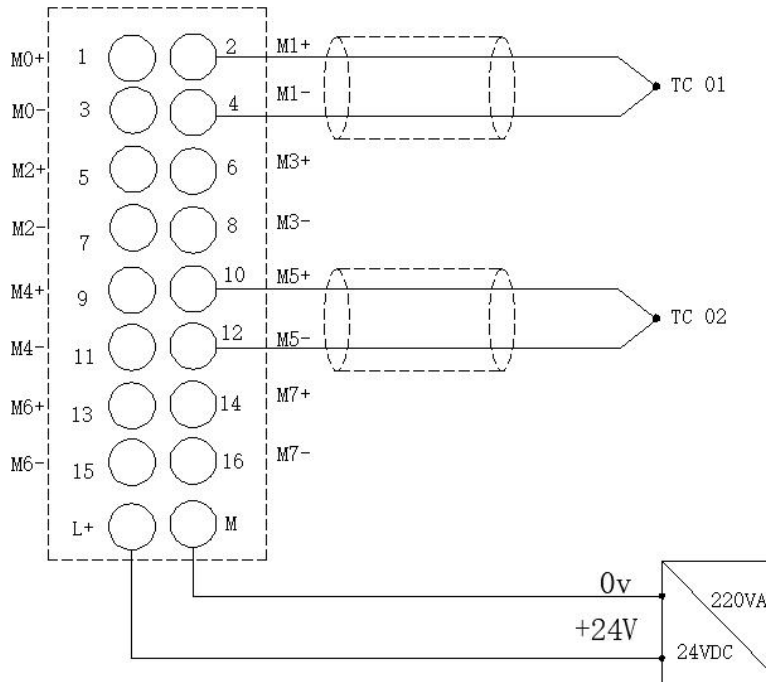
接线图
