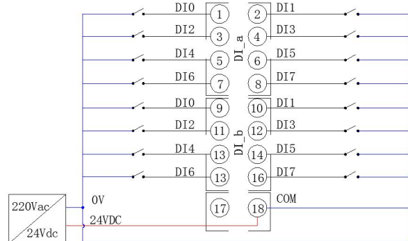
DI 接线图 (NPN)
