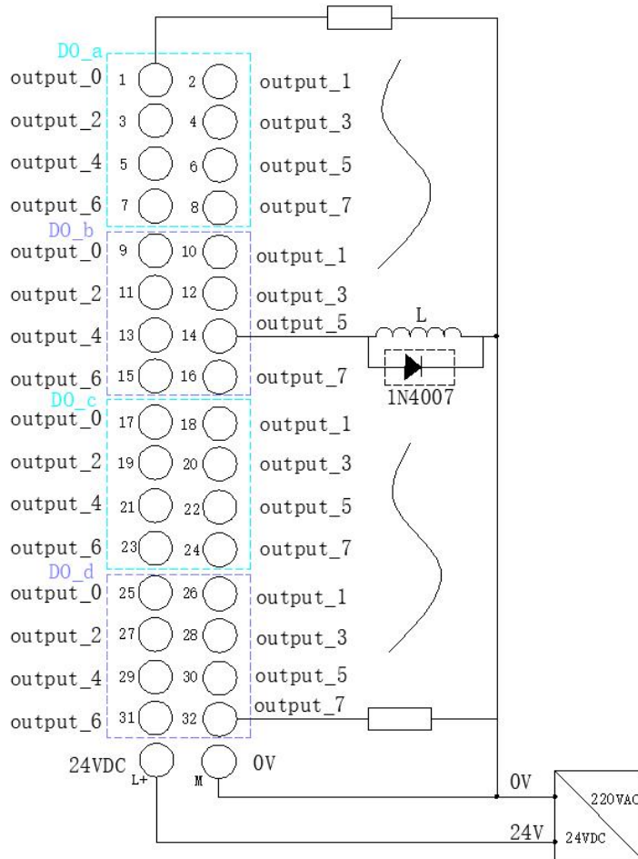
接线图
