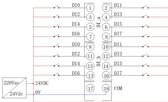
DI 接线图 (PNP)
