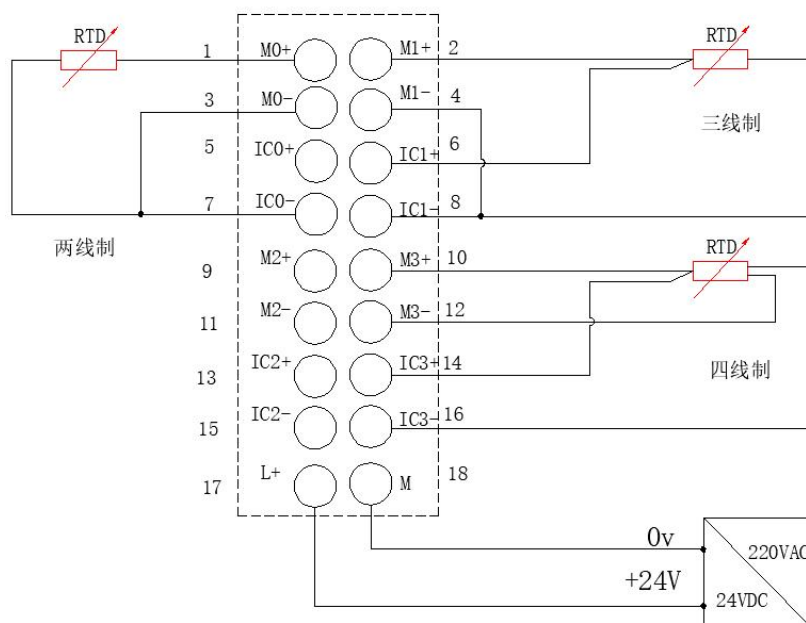
接线图
