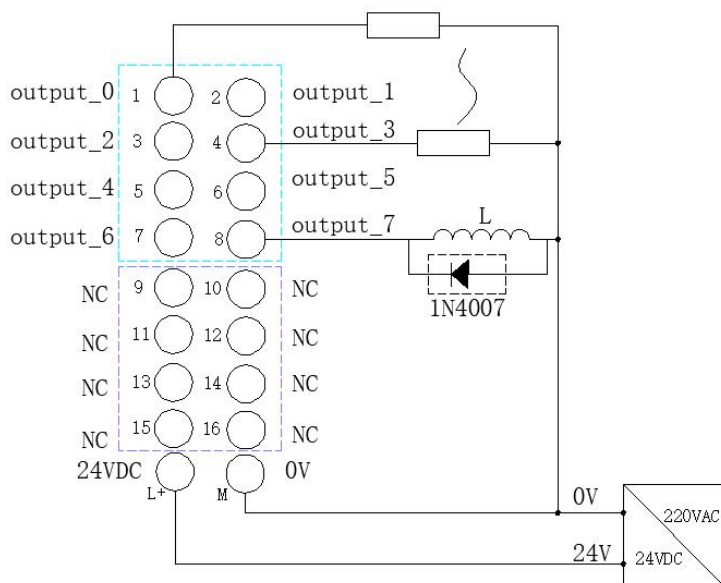
接线图
