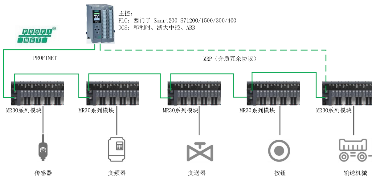
图 13-1 通讯连接图
