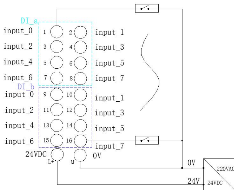
接线图
